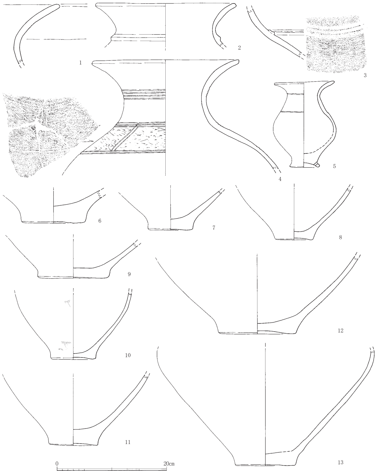
第15图 18号土坑出土遺物実測图1 (1/4)
