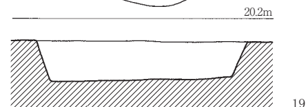
第25図 17・19号土坑 実測図 (1/40)
